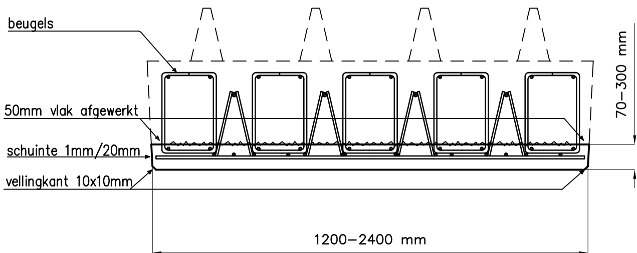
doorsnede Kolomkop met beugels
