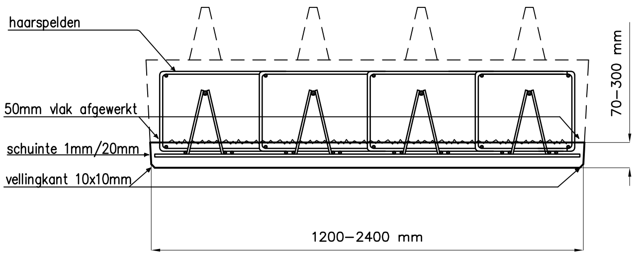
doorsnede Kolomkop met haarspelden
