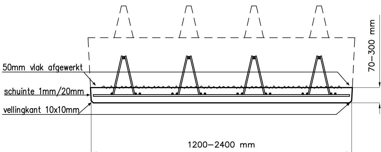
doorsnede Kolomkop
