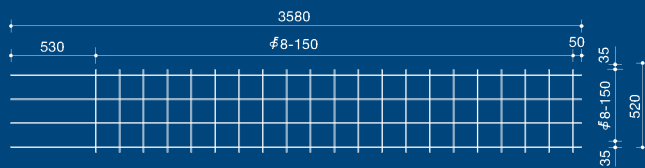
Wapeningsmat voor funderingsstrook van 600 mm breed
